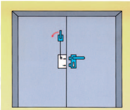
Bild 4: Paniktreibriegel an zweiflügeliger Notausgangstür
