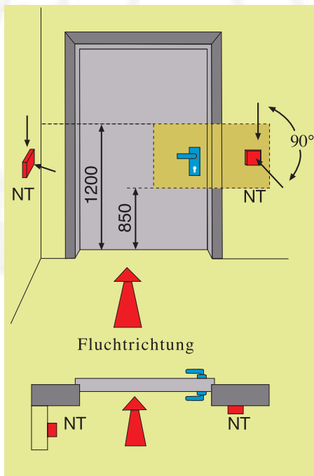
Bild 9: Anbringung der Nottaste
