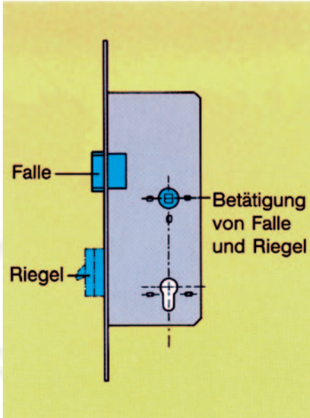
Bild 2: Panikschloss
